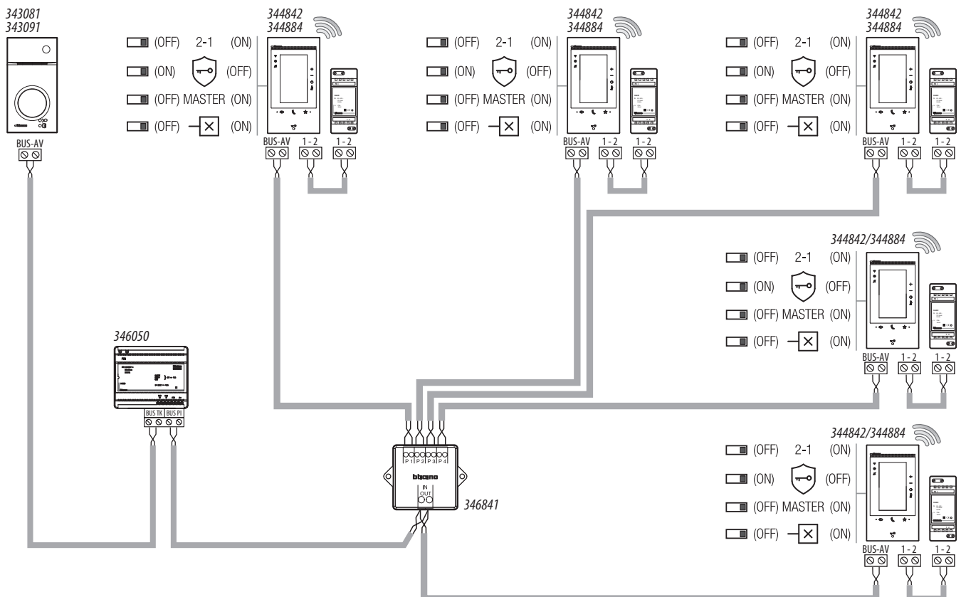
SCHEMA 7 - ESEMPIO SCHEMA MONOFAMILIARE CON 5 CLASSE 300EOS WITH NETATMO
