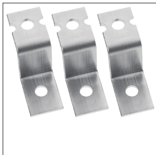
S-2AV
