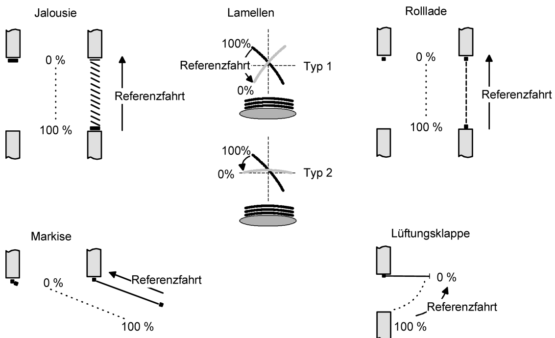
Bild 12: Referenzfahrt
