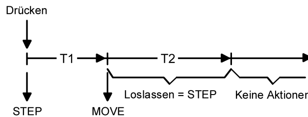
Bild 34: Bedienkonzept "Kurz-Lang-Kurz"
