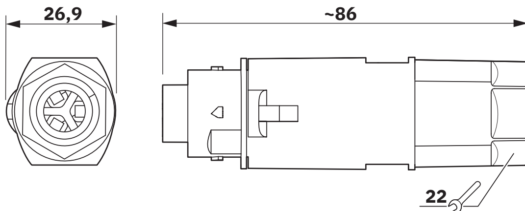
Disegno quotato
