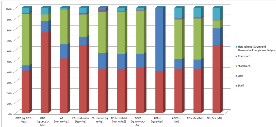
Abbildung 10: Prozentuale Anteile ausgewählter Komponenten der Herstellung und der Transporte im Produktionsstadium anhand ausgewählter Umweltwirkungskategorien (Gitterrinnensystem)
