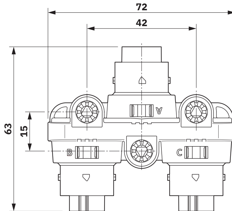
Disegno quotato
